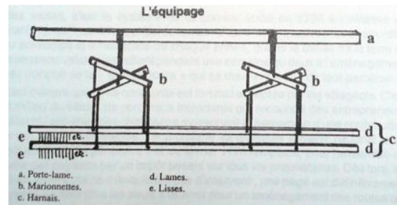
Schéma de « l'équipage » d'un métier à tisser.
