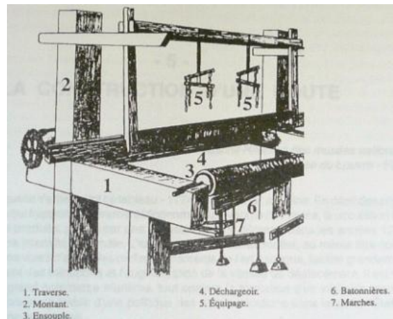
Structure générale d'un métier à tisser.
